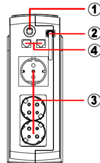
Panel del paquete VFD 1000
